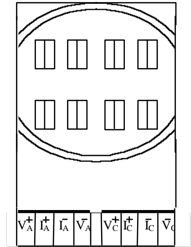
Form 5S (SWRWS5) wiring diagram
